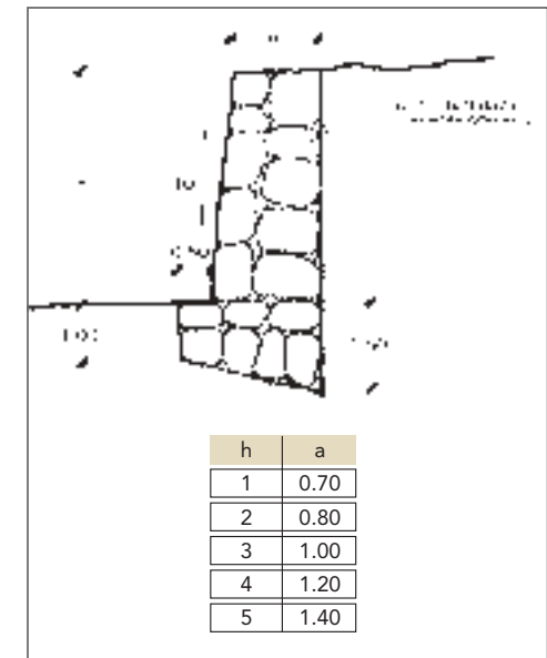
• Sección tipo de escollera hormigonada.
