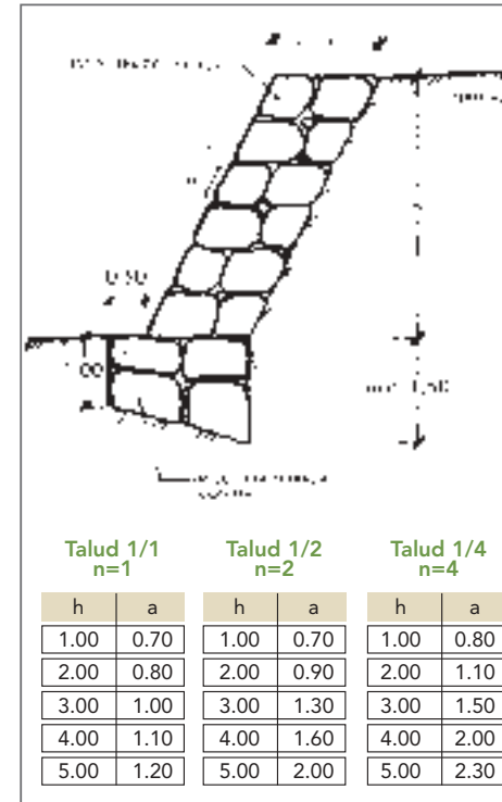
• Sección y características de un muro de escollera convencional.
