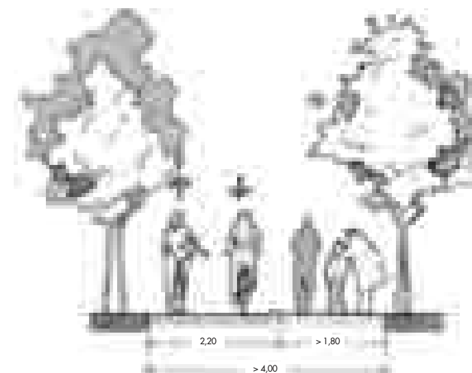
• Senda bici sin segregación entre peatones y ciclistas.
