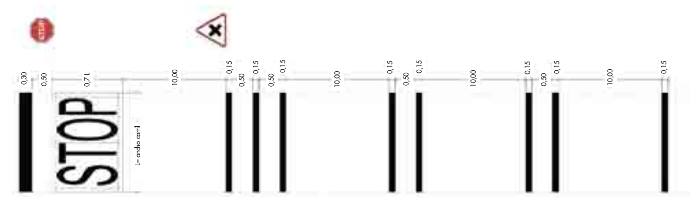
• Caso 1: señalización de cruce entre una vía ciclista y una vía motorizada de alta intensidad de tráfico con prioridad de paso.
