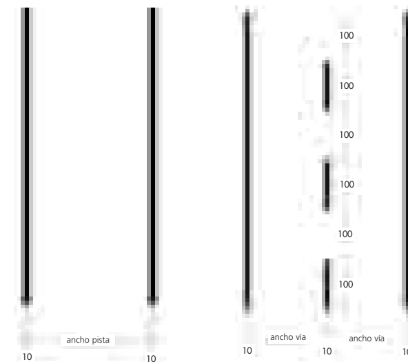
• Delimitación de calzada en pistas bici, acera bici y sendas bici segregación de banda ciclista.
