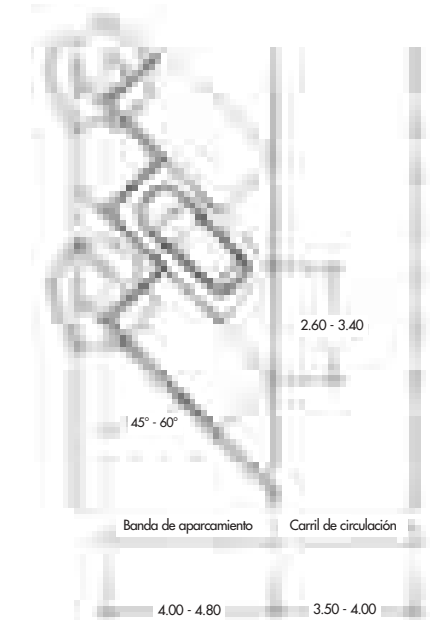
• Espacio de aparcamiento en batería (en ángulo).
